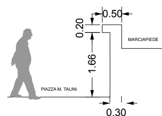
SEZIONE A-A'
